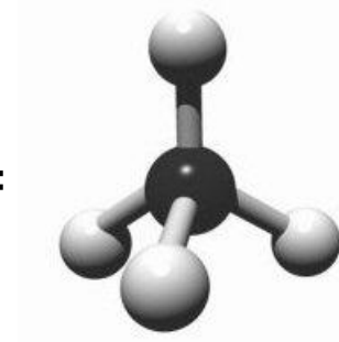
Metan
